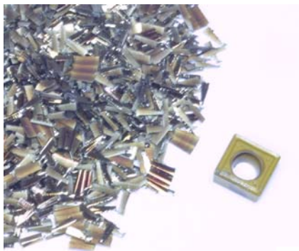
SCGT 060204 EN DC15 Material: 1.2343 / dry
