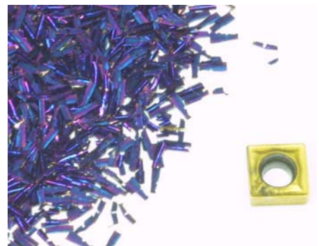
SCMT 060204 EN DC15 Material: 1.2343 / dry
